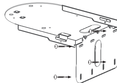
3. 將 VC-AC08 底座鎖固於牆面上
