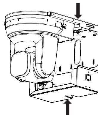
7. 整理線材，扣上板金蓋
