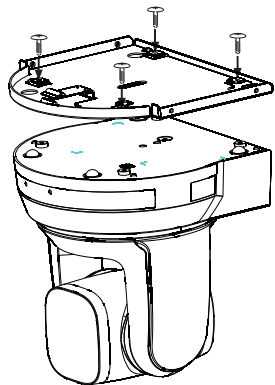
1. 將攝像機鎖固於拖盤上
